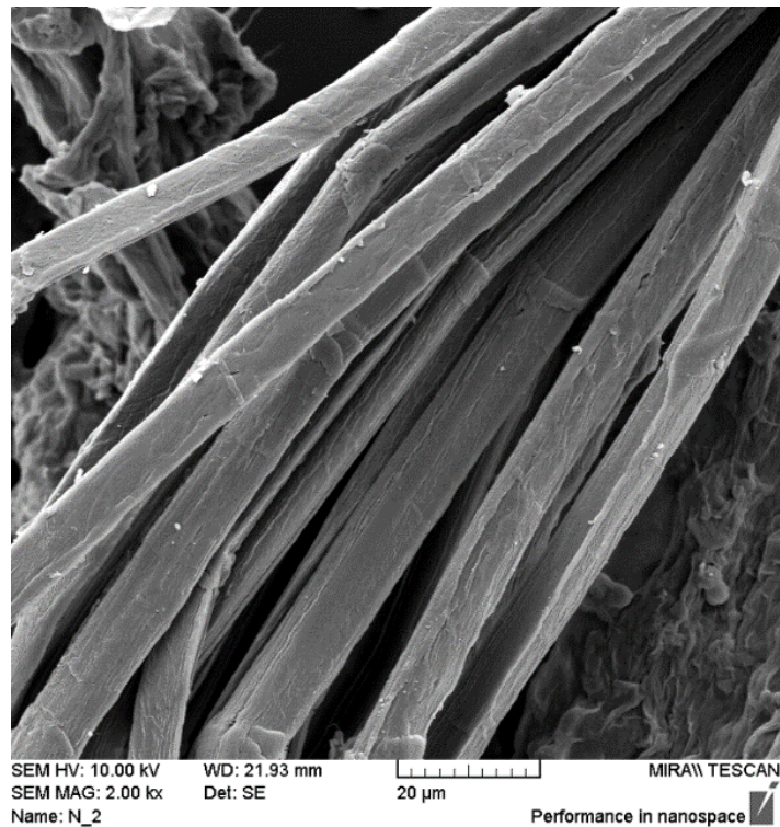
Slika 2.3.4. Morfološka karakterizacija uzoraka vlakna brnistre na Mira LMU FE-SEM, Tescan mikroskopu
